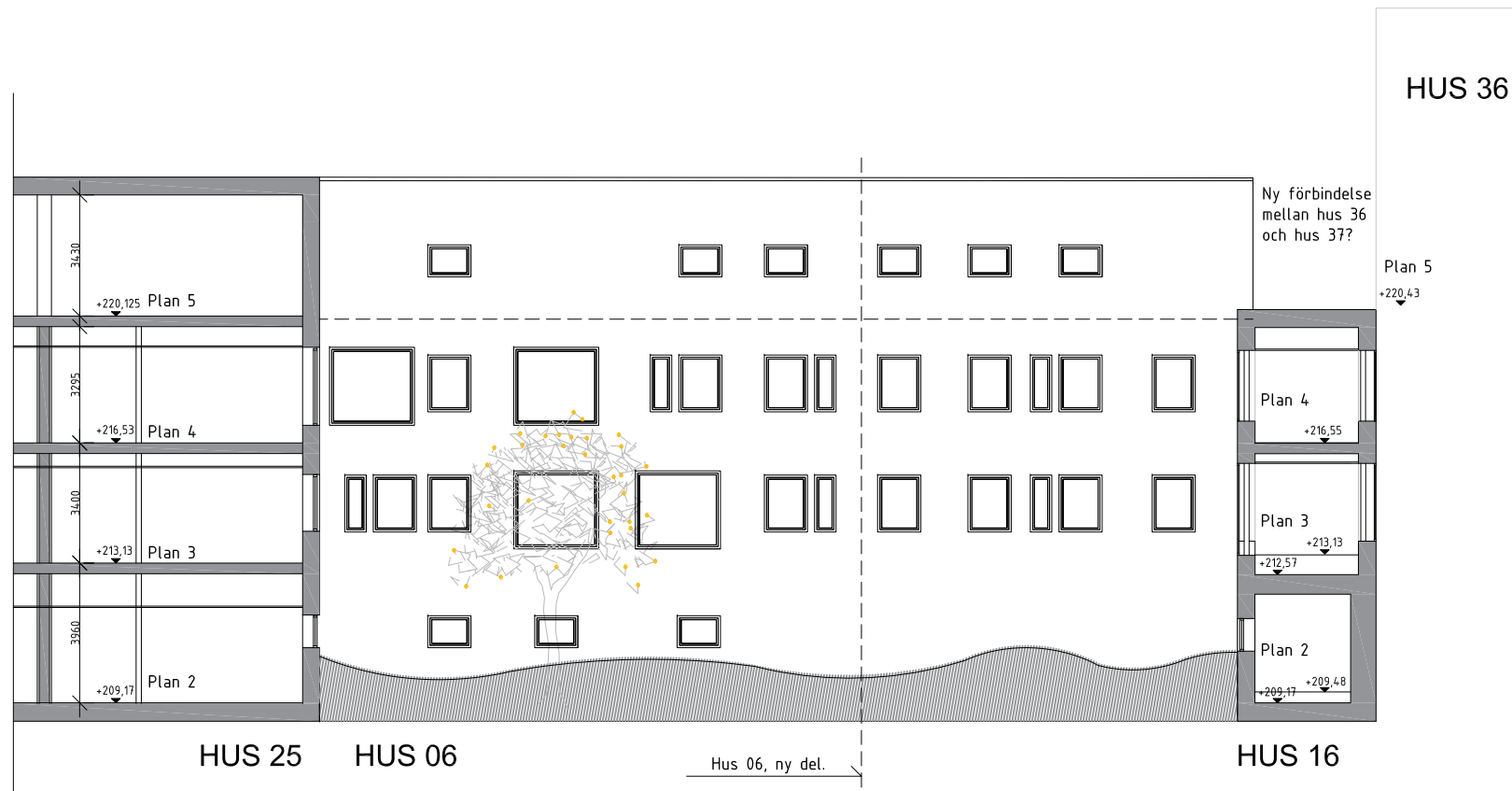
Ny fasad mot innergård, NORR
